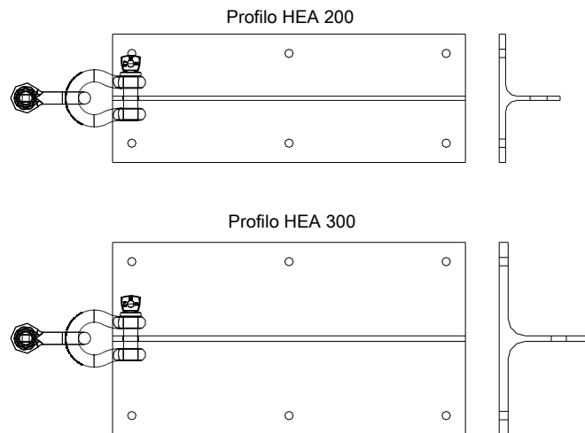
Figura 4.96 Dettaglio forature su profili HEA200 e HEA300.
