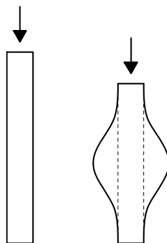
Figura 4.88 Tipico dissesto di pareti "a sacco" sovraccaricate.
