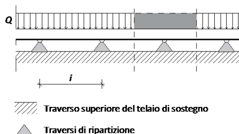
Figura 4.48 Schema dei carichi di progetto ("T"). Il carico Q del solaio viene riportato sui telai paralleli attraverso dei traversi di ripartizione.
