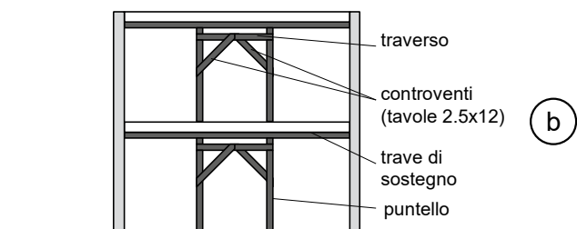
Sezione trasversale
