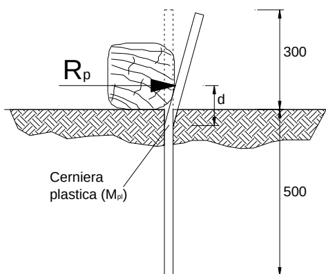
Figura 4.93 Schema meccanismo di collasso per configurazione picchetto Singolo o Doppio (misure in mm).
